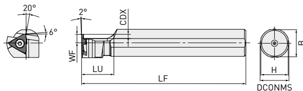
Portautensile sinistro
